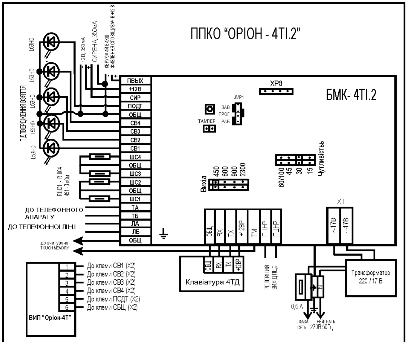
Рисунок А.1 - Схема електрична підключення
